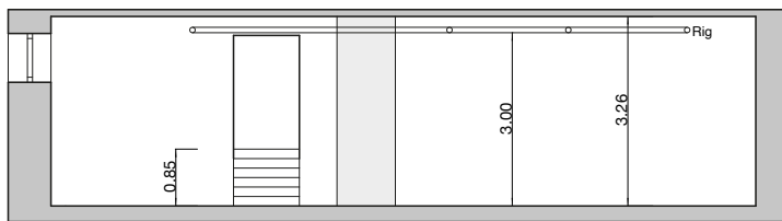
Schnitt A-A
